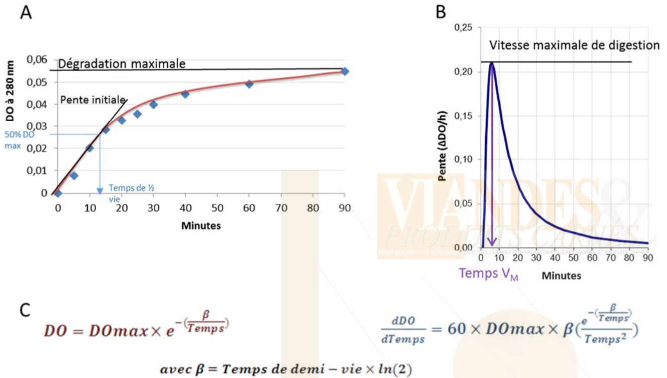
Figure 1 : Allure de la courbe de digestion (A), paramètres de digestion (B après calcul de la dérivée de la courbe de la Figure 1A) et équations correspondantes (C)
