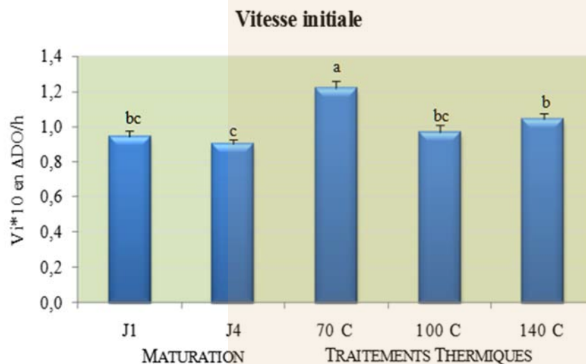
Figure 2 : Vitesse initiale de digestion in vitro à la pepsine en fonction de la durée de maturation et de la température de cuisson de la viande
