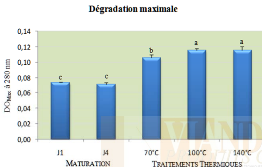
Figure 3 : Effets de la maturation et des traitements thermiques sur l'hydrolyse maximale
